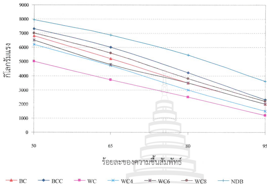
ภาพที่ 17 การเปลี่ยนแปลงของค่าความต้านทานการกดของภาชนะบรรจุในแต่ละสภาวะทดสอบที่ความขึ้นสนิมพัทธ์ร้อยละ 50 65 80 และ 95 และอุณหภูมิ 10 องศาเซลเซียส
