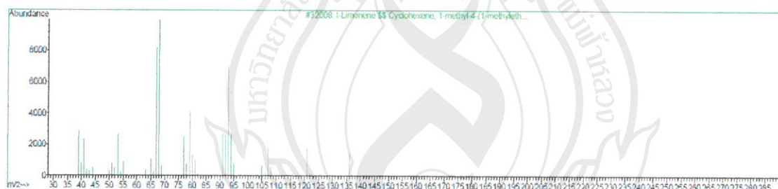
ภาพที่ 4-5 Mass spectrum มาตรฐานของ l-limonene
