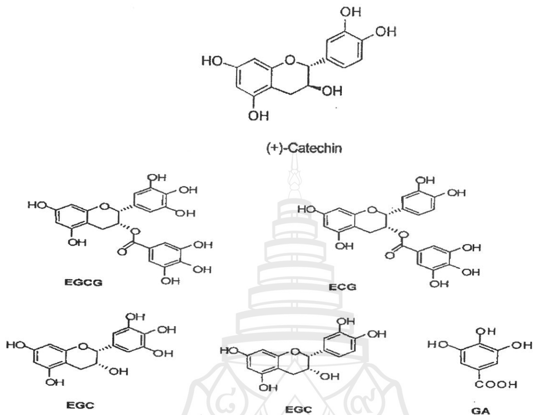
รูปที่ 2.2 โครงสร้างของสารประกอบคาเทชินและกรดแกลลิก, (-) -epigallocatechin-3-gallate (EGCG), (-)-epigallocatechin (EGC), (-)-epicatechin-3-gallate (ECG), (-)-epicatechin (EC) และ gallic acid (GA) (ที่มา Cabrera และคณะ 2006)
